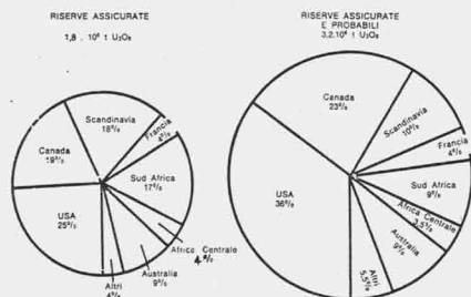
Fig. 5 - Distribuzione geografica delle riserve di uranio. Categoria di prezzo < 15 $/lb U 3 O 8 (inizio 1974)
